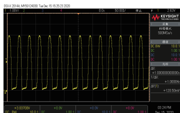
▲ 常规负载出现自激现象
