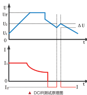
▲ DCIR测试原理图
