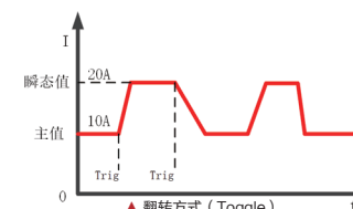
▲ 翻转方式 (Toggle)
