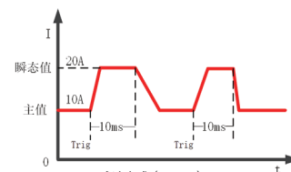
▲ 脉冲方式 (Pulse)
